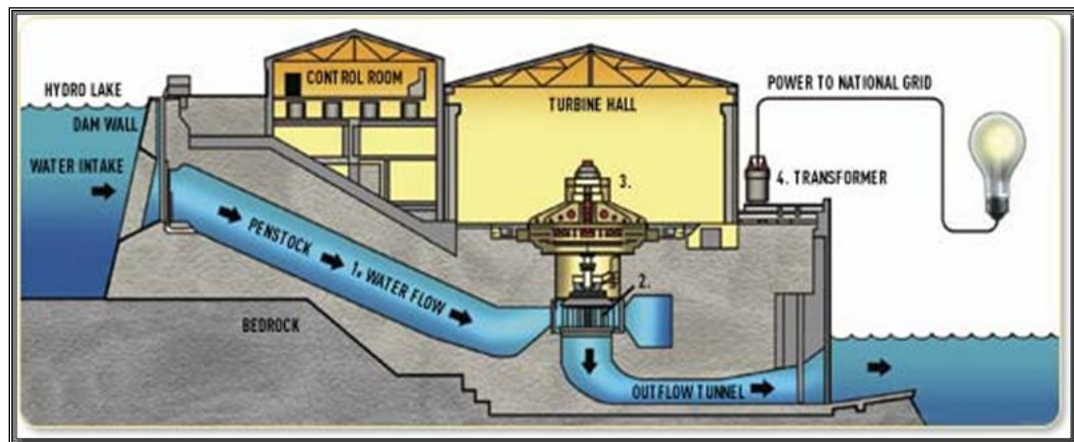
Gambar 1. Bentuk PLTA
