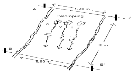
Gambar 5. Langkah Pengukuran kecepatan aliran sungai
