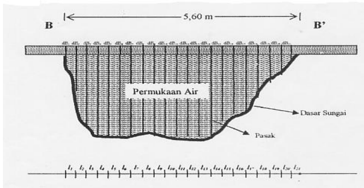
Gambar 4. Pengukuran Pada Hilir Sungai
