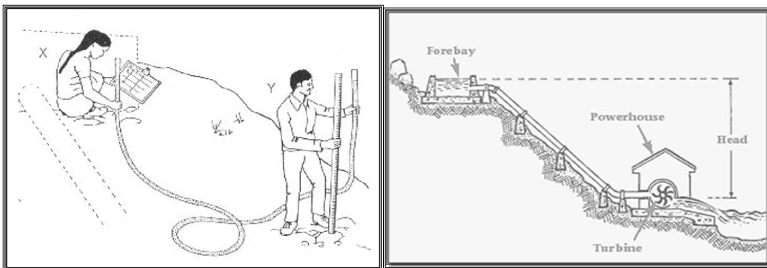
Gambar2. Pengukuran debit dan tinggi jatuh air
