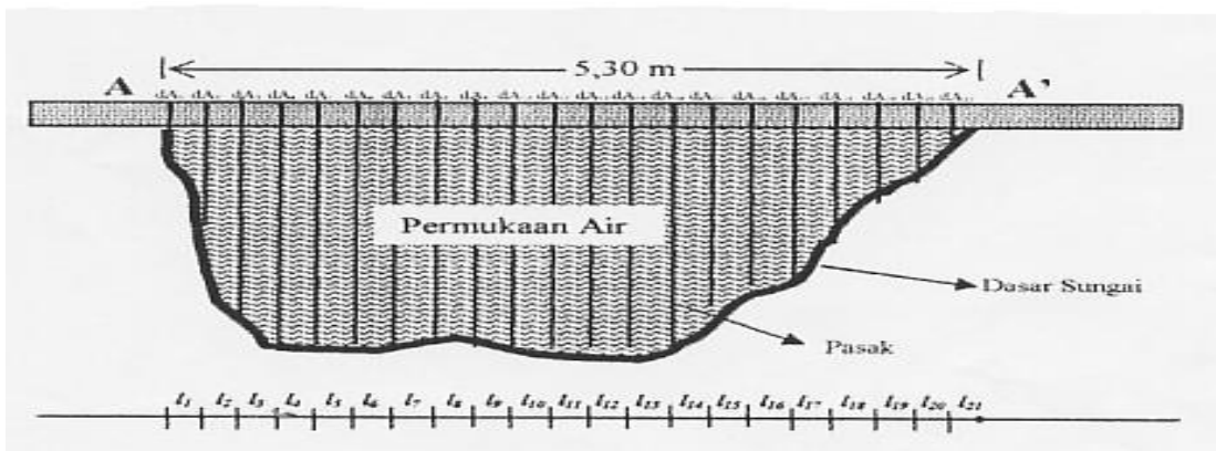
Gambar 3. Pengukuran kedalaman Sungai
