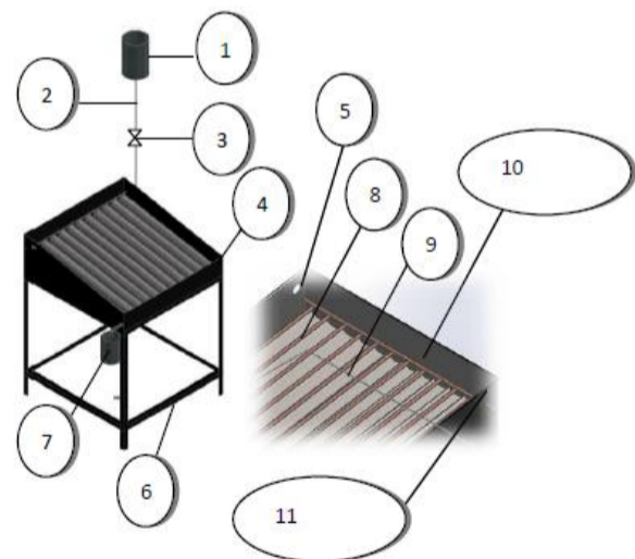
Gambar 3 Bagian – bagian solar kolektor Keterangan gambar :
