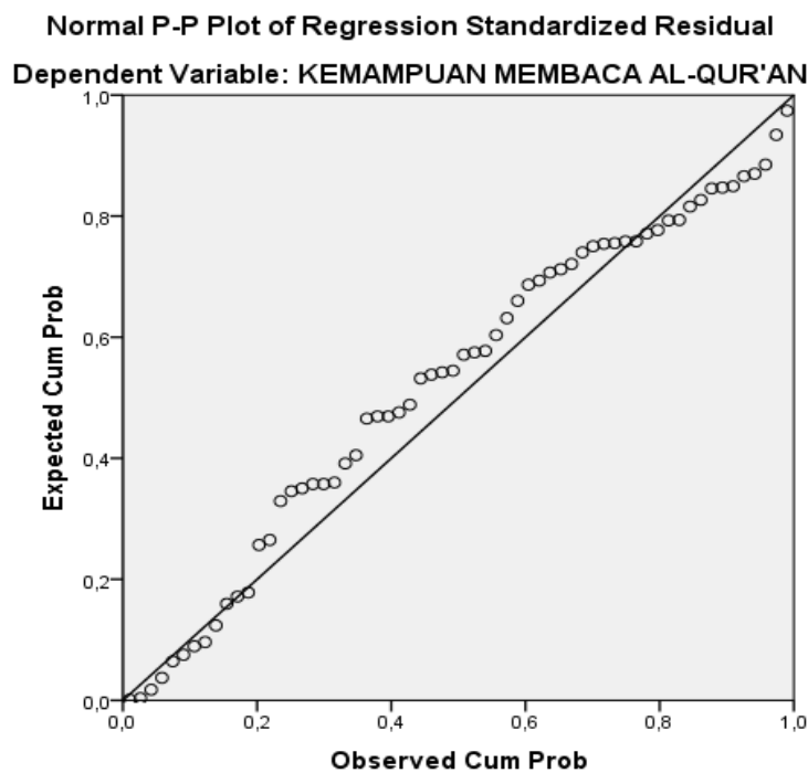
Gambar 1. Uji Normalitas Data
